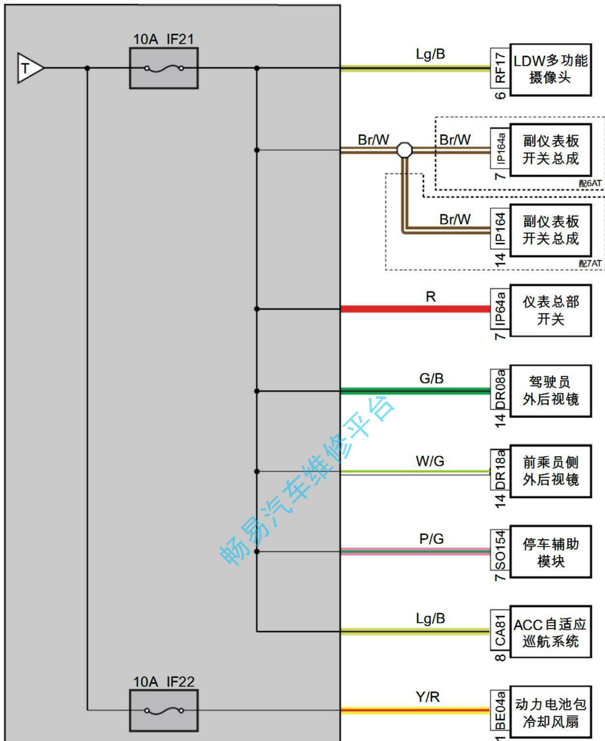
室内保险丝、继电器盒电源分布图 (续4)
