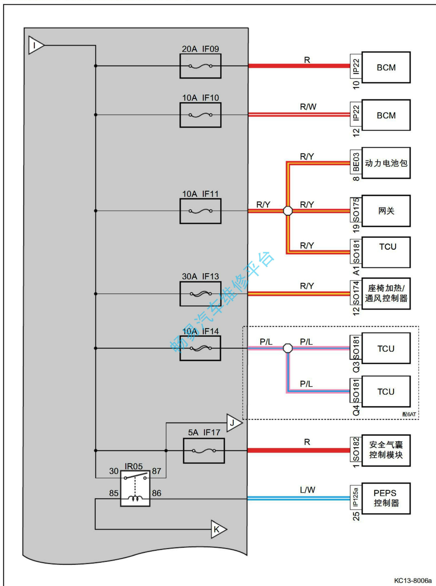
室内保险丝、继电器盒电源分布图 (续1)
