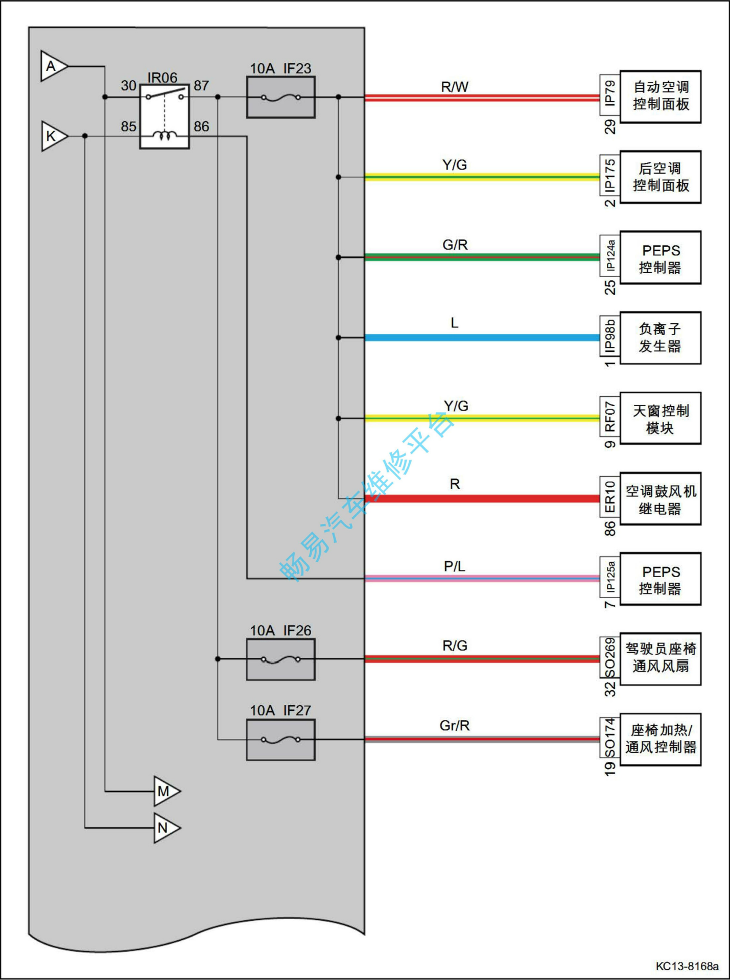
室内保险丝、继电器盒电源分布图 ( 续5 )
