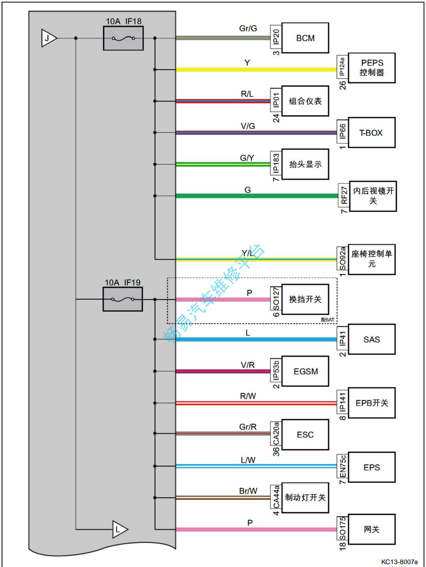
室内保险丝、继电器盒电源分布图 (续2)
