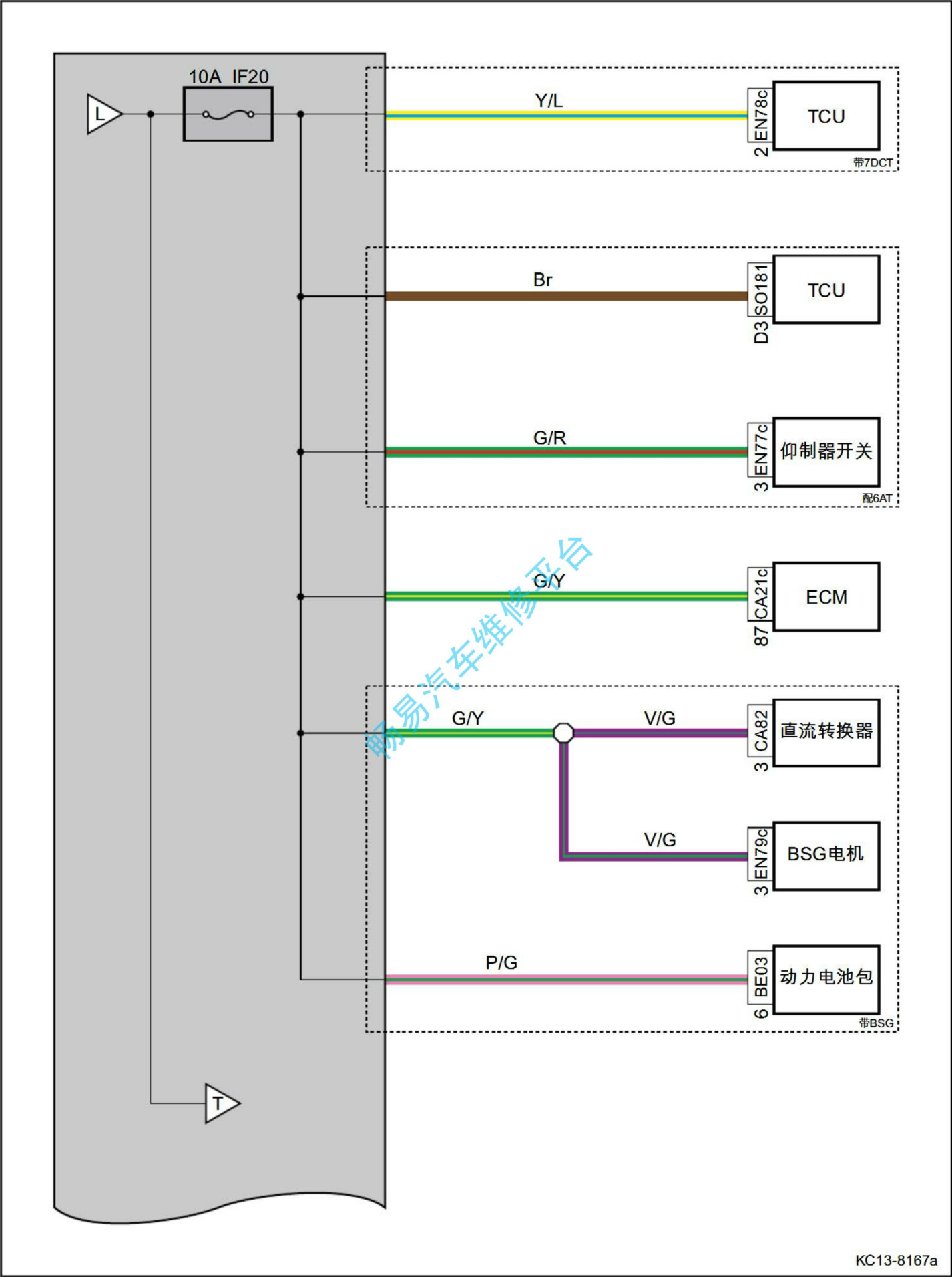
室内保险丝、继电器盒电源分布图（续3）
