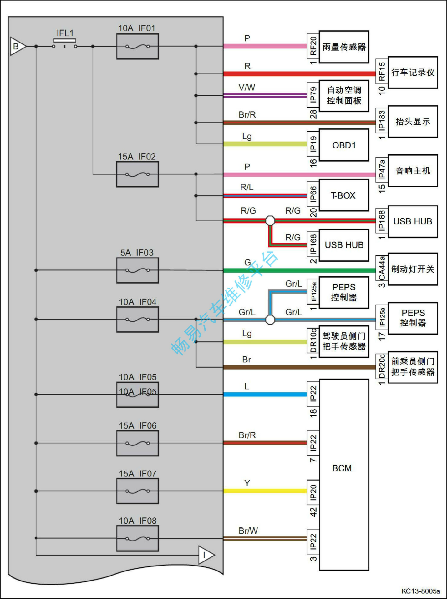
室内保险丝、继电器盒电源分布图
