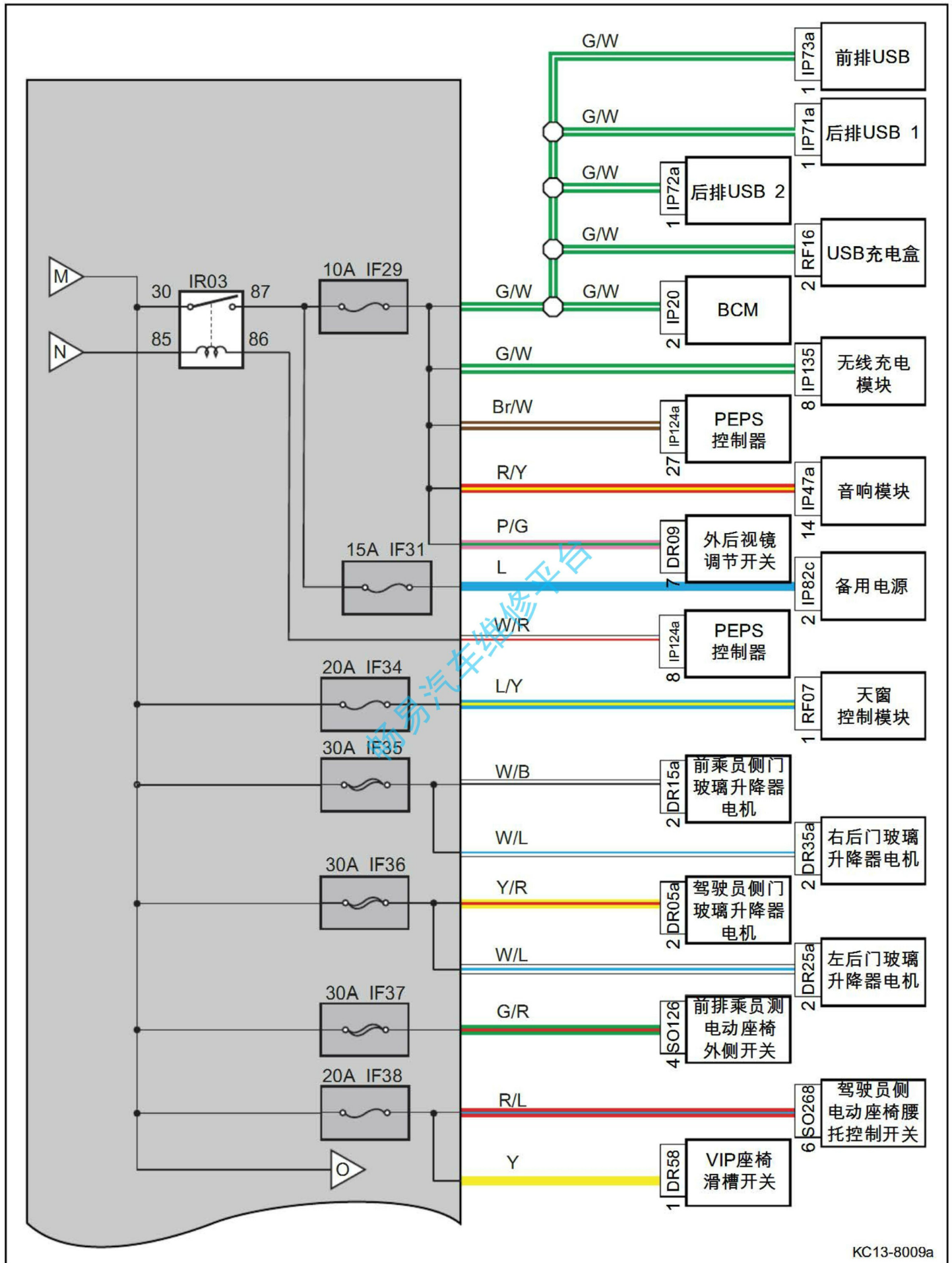
室内保险丝、继电器盒电源分布图 (续6)
